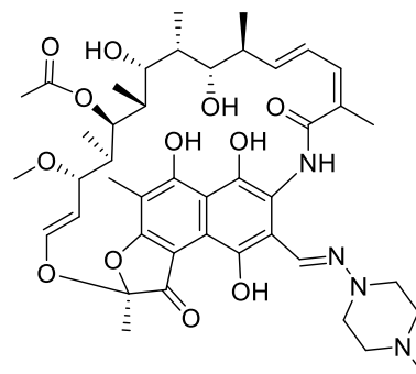
Rifampicin
