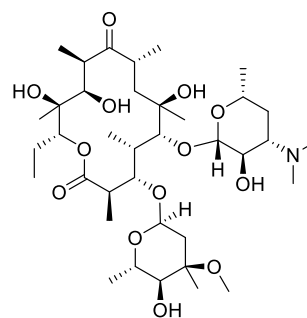
Erythromycin A
