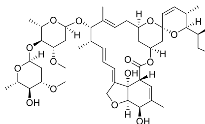
Avermectin B1a
