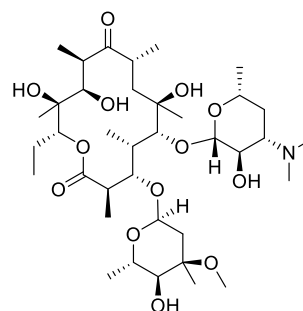
Erythromycin A
