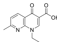
Nalidixic acid
