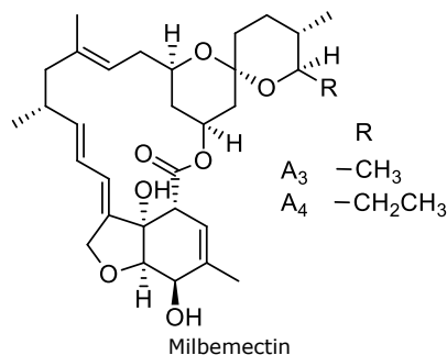
Milbemectin
